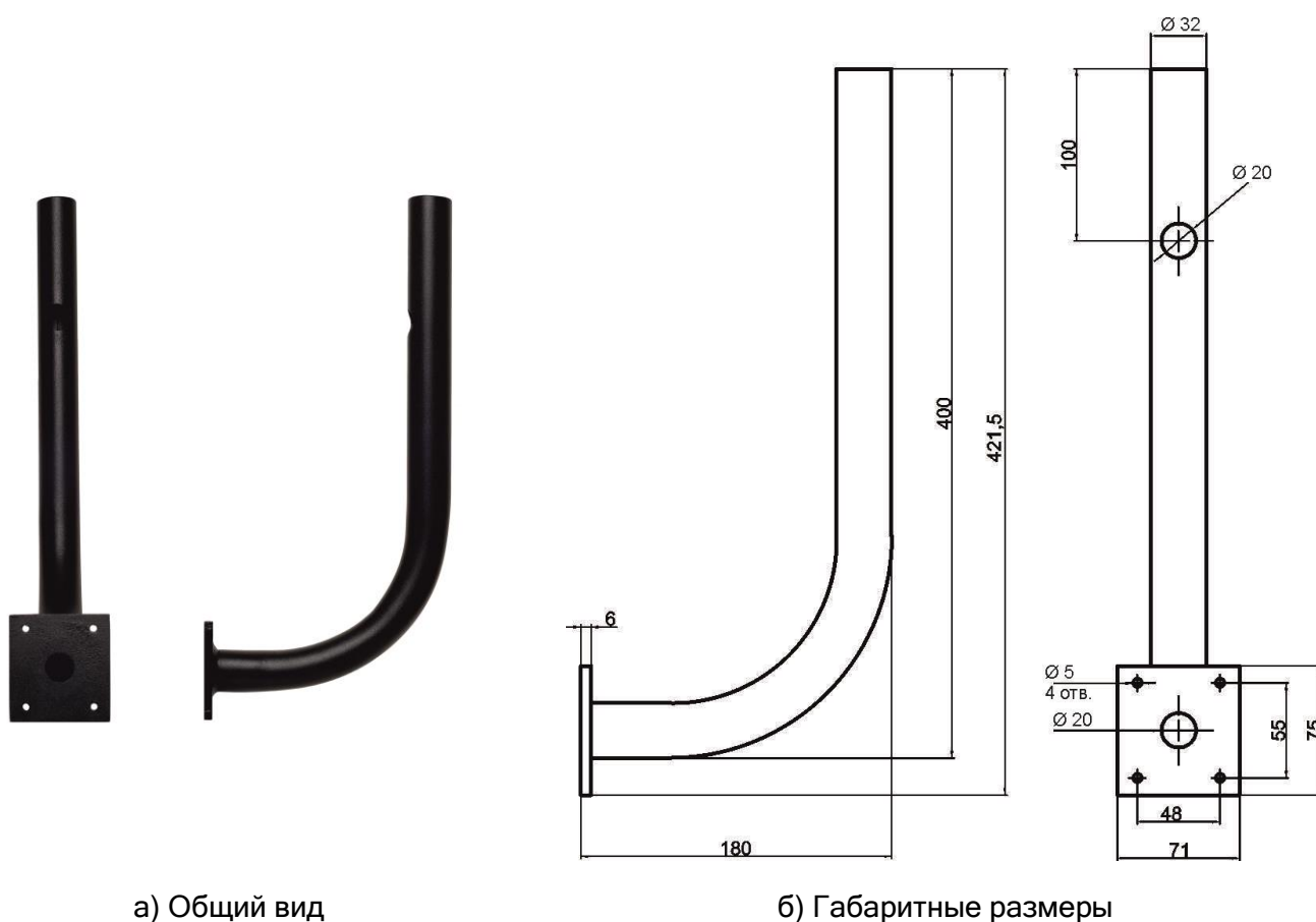
Рисунок 1 - Общий вид кронштейна с габаритными размерами
